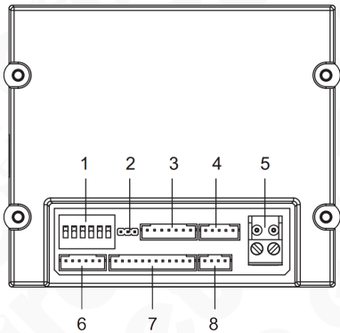
Fig. 14. Camera module terminals
